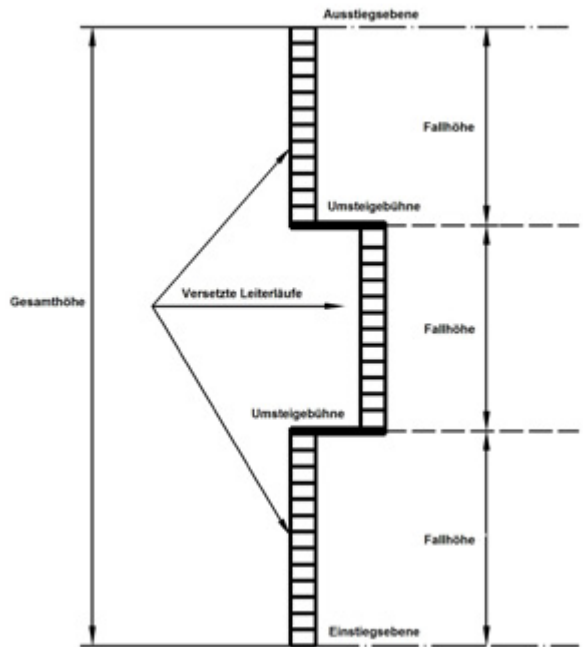
Abb. 5 Mehrzügige Steigleiter
