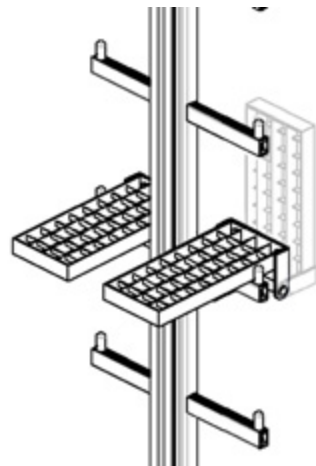
Abb. 7 Bewegliche Ruheebene (zweiteilig)
