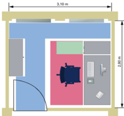
Abb. 13: Zellenbüro/Einzelbüro Beispiel 1 (Quelle: VBG Hamburg [ www.vbg.de ])
