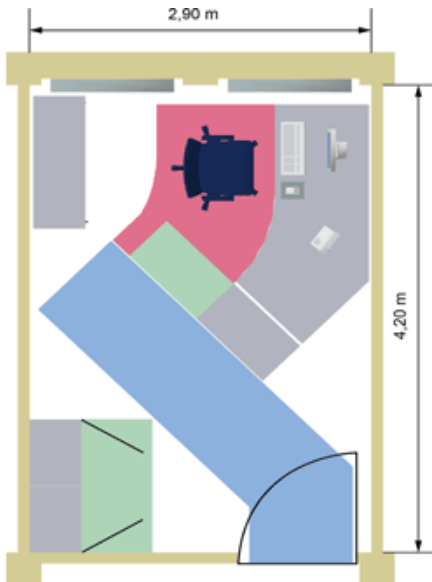
Abb. 14: Zellenbüro/Einzelbüro Beispiel 2 (Quelle: VBG Hamburg [ www.vbg.de ])
