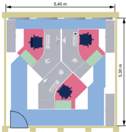
Abb. 16: Drei-Personen-Büro (Quelle: VBG Hamburg [ www.vbg.de ])
