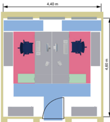
Abb. 15: Zwei-Personen-Büro (Quelle: VBG Hamburg [ www.vbg.de ])
