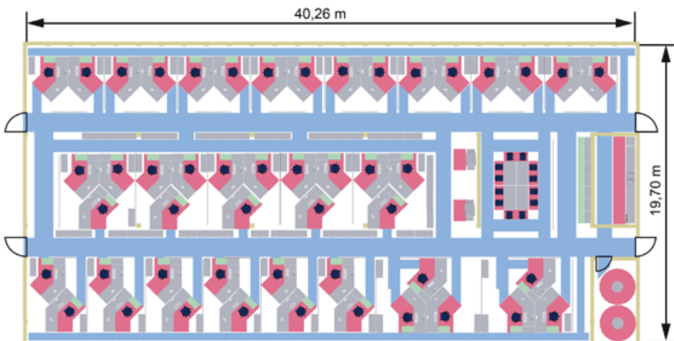
Abb. 19: Großraumbüro (Quelle: VBG Hamburg [ www.vbg.de ])
