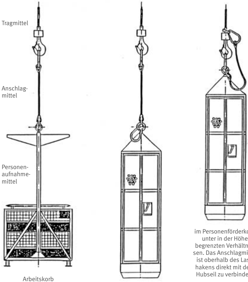
Personenförderkorb im Normalfall
