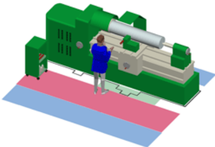
Abb. 12: 3D-Ansicht (Quelle: VBG Hamburg [ www.vbg.de ])
