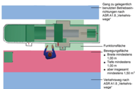
Abb. 11: Grundriss (Quelle: VBG Hamburg [ www.vbg.de ])
