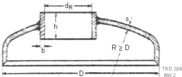
Bild 2. Gewölbter Flammrohrboden mit Verstärkungsring
