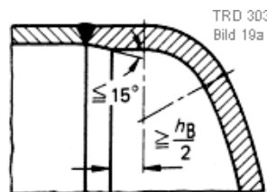
Ausführung b
