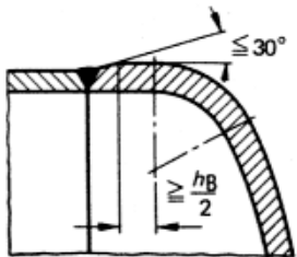
Ausführung b
