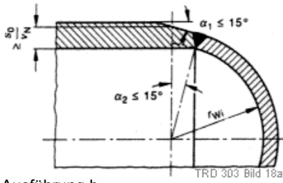
Ausführung b
