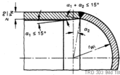
Bild 19. Anschluß eines gewölbten Bodens an Zylinder mit kleinerer Wanddicke
