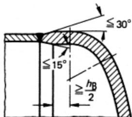
Ausführung c
