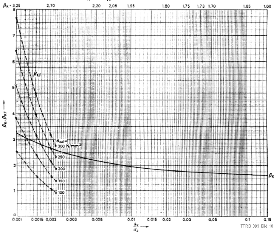
Bild 16. Berechnungsbeiwerte \beta_K und \beta_{KF} für tiefgewölbte Böden
