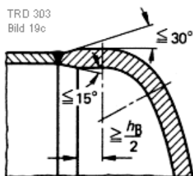
Ausführung c
