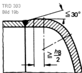
Ausführung c
