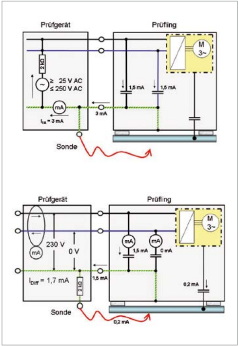
Beispiel Abb. 5.11 und 5.12 Die Schutzleiterstrommessung erfolgt über den PE-Kontakt der Prüfsteckdose, die Berührungstrommessung über die Sonde. Sind beide Messpfade, z. B. beim Differenzstrommessverfahren oder beim Ersatz-Ableitstrommessverfahren, aktiv und ist die Sonde von den vorhergehenden Messungen des Schutzleiterwiderstands oder des Isolationswiderstands noch angeklemmt, dann gibt die Messwertanzeige die Summe aus beiden Strömen an, ohne dass der Prüfer dieses erkennen kann.
