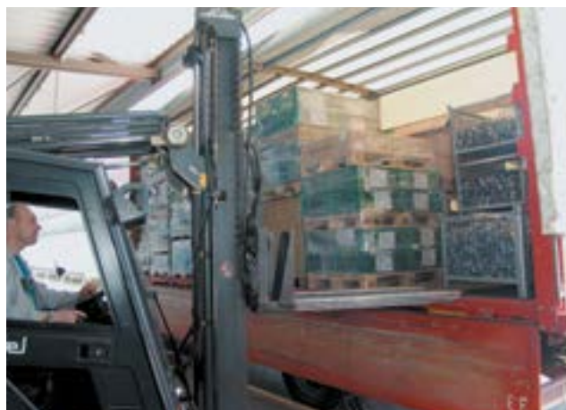
Bild 8-5: Beim Be- und Entladen von Fahrzeugen sind diese immer gegen Wegrollen zu sichern. Das heißt, der Gang ist einzulegen, die Feststellbremse anzuziehen und der Unterlegkeil unterzulegen
