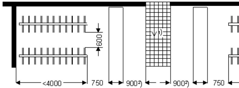
Abgabegarderoben, zweibündig mit Bügelgestell
