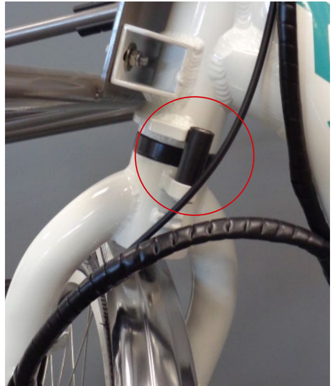
Abb. 22 Lenkungseinschlagbegrenzer
